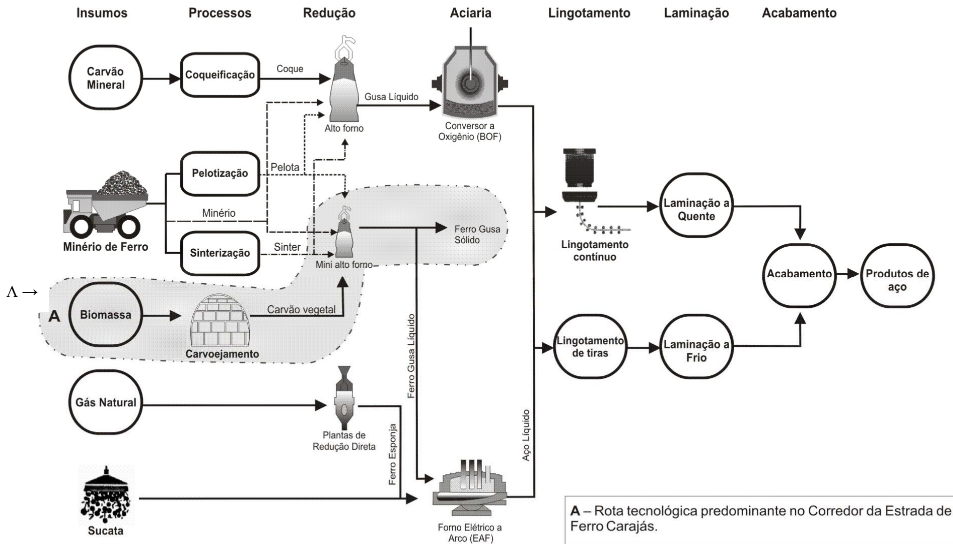
Figura 2: Representação esquemática das principais rotas tecnológicas utilizadas para a produção de aço
