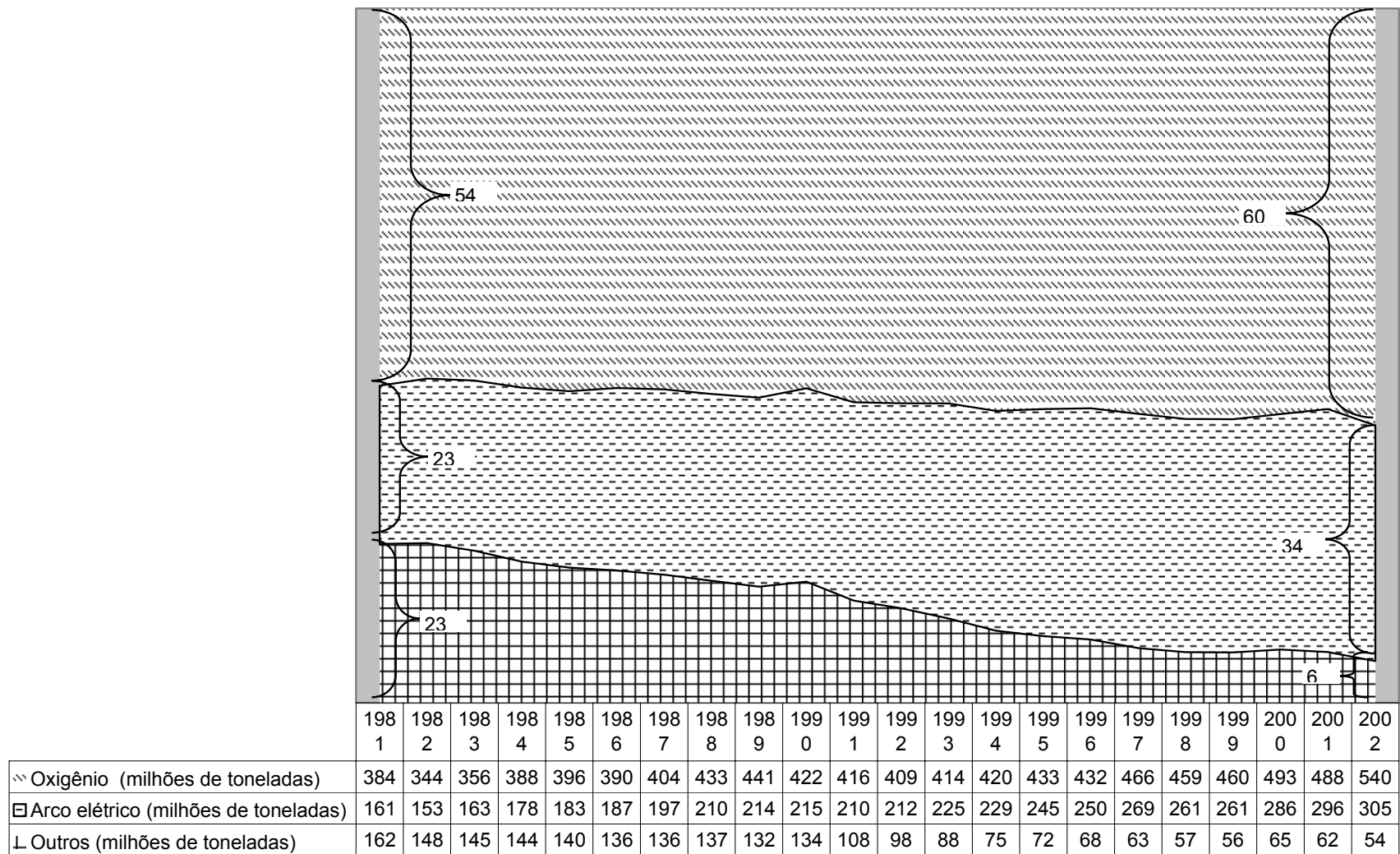
Figura 1: Produção mundial de aço bruto por processo de aciaria.
